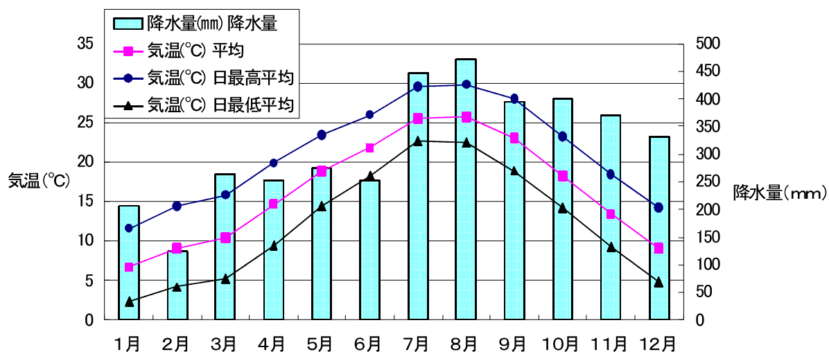
平成21年中降水量と月別平均気温
