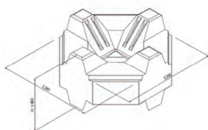
オルサーブロック 1 段積み
