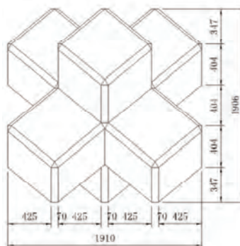
六脚ブロック
