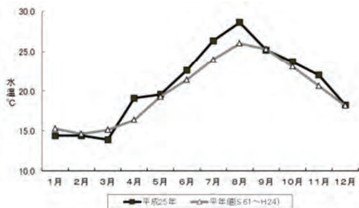
古里養殖場(水温)
