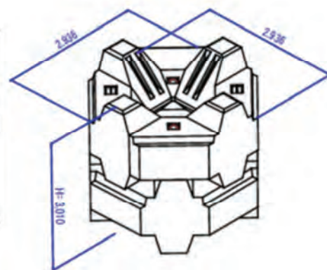
オルサーブロック 2 段積み
