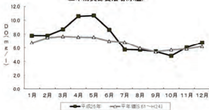
古里養殖場(溶存酸素)
