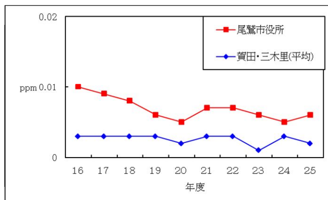
図-3.1.1.3 二酸化窒素の経年変化
