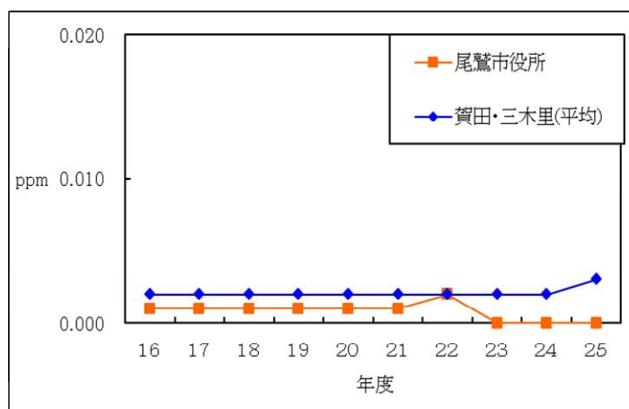
図-3.1.1.2 二酸化硫黄の経年変化
