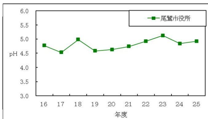
図-3.1.1.4 降水の pH の経年変化
