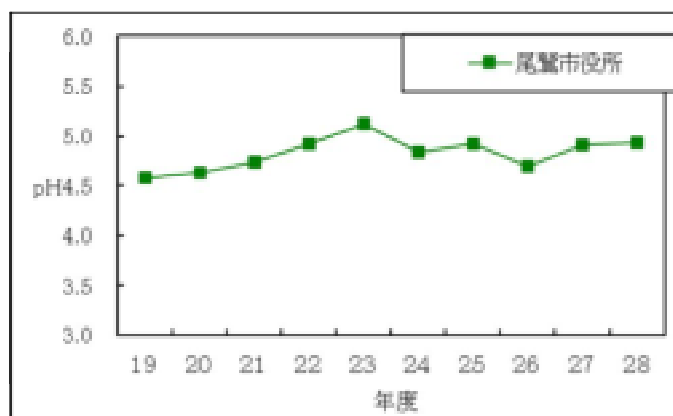
図-3.1.1.4 降水の pH の経年変化
