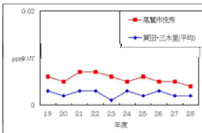
図-3.1.1.3 二酸化窒素の経年変化
