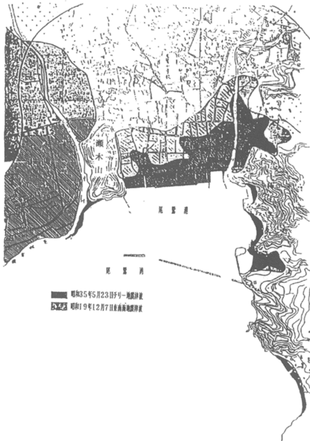
②東南海地震津波とチリ地震津波の浸水区域比較図（尾鷲地区）
