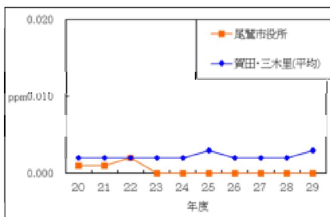
図-3.1.1.2 二酸化硫黄の経年変化
