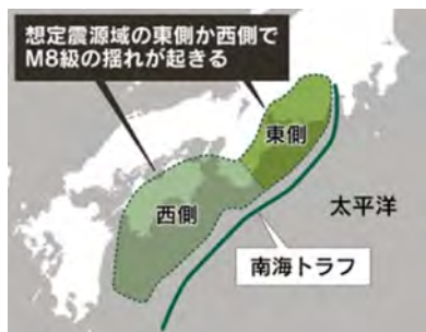
南海トラフ巨大地震の「半割れ」ケース
