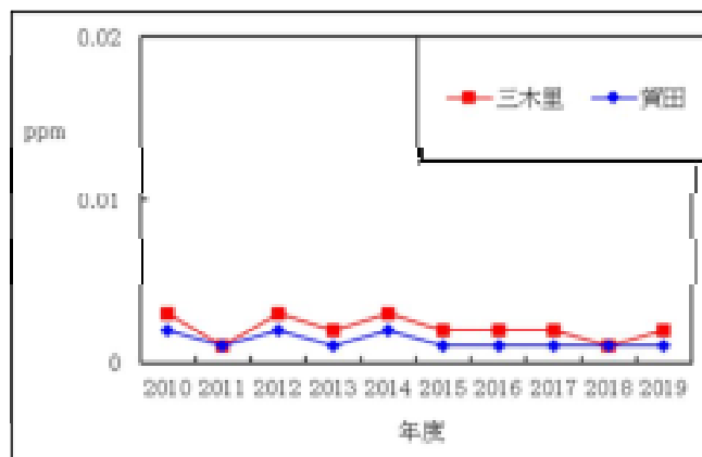
図-3.1.1.3 二酸化窒素の経年変化
