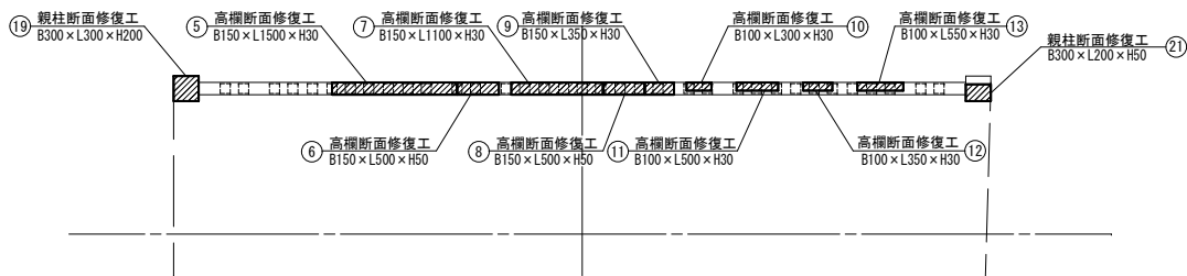
平面図
