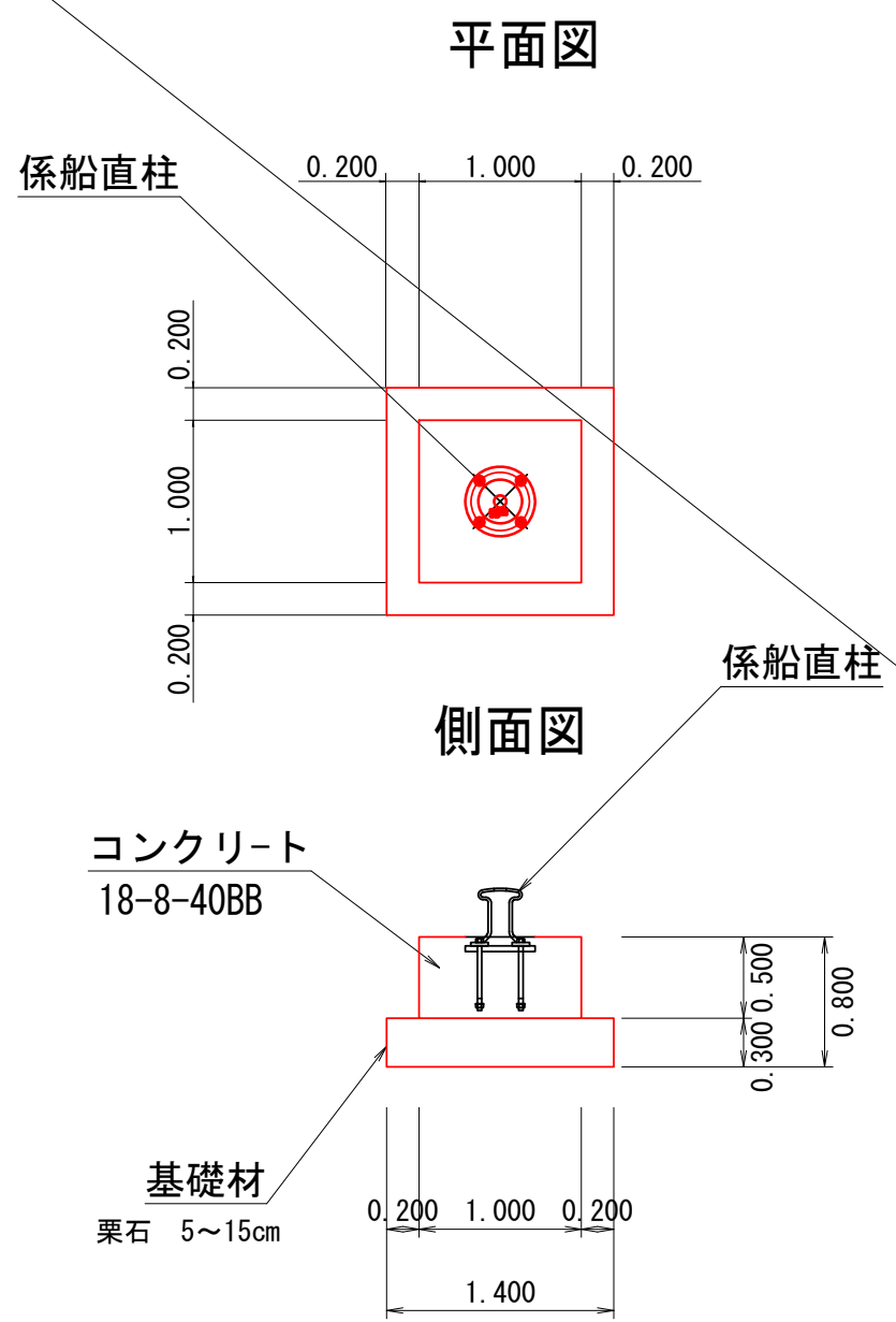
係船直柱詳細図 (参考) S=1:50
