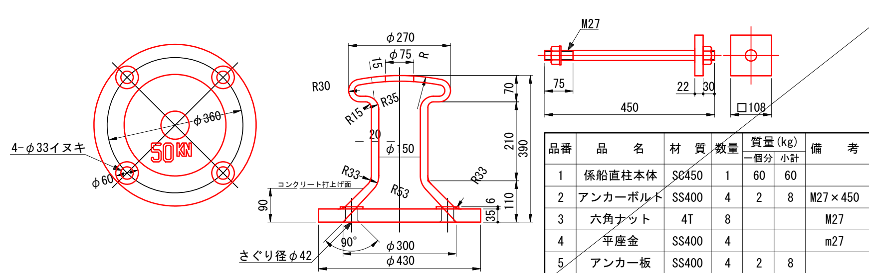
係船直柱詳細図 (参考) S=1:10
