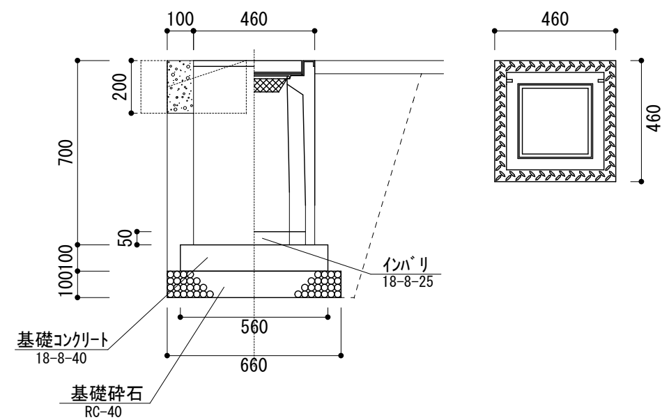
柵工③ 詳細図 (PU柵口250×250A H=550相当品)
