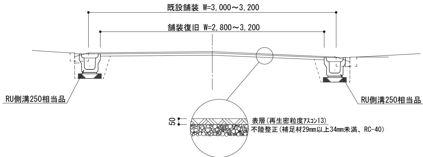
側溝工 標準断面図②
