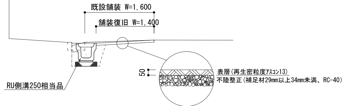
側溝工 詳細図 (RU側溝250用 相当品)
