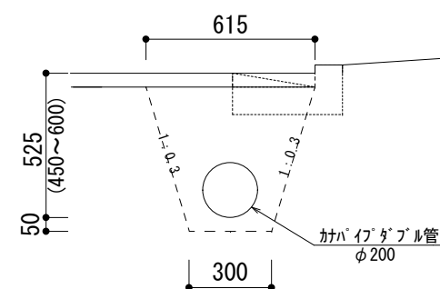
暗渠排水管工 詳細図
